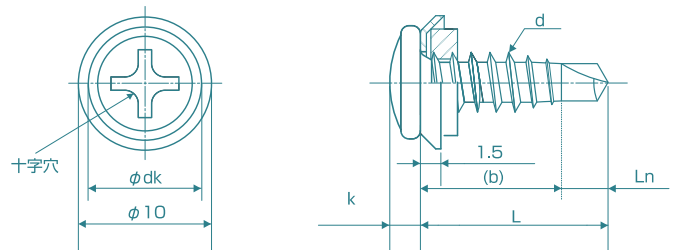
PSPタイプ (座金・パッキン付)
